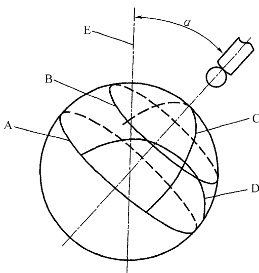
图 4 检测球上四个目标扫描平面
