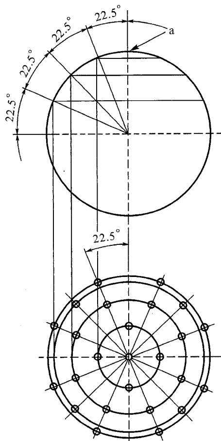
图1 探测误差测量点分布
