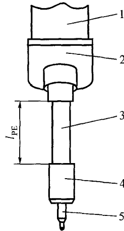
图 6 垂直位置时转向测头系统
